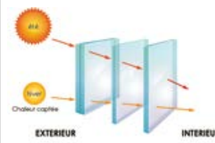
TRIPLE VITRAGE 52 À 68 MM 1 FACE FEUILLETÉE
